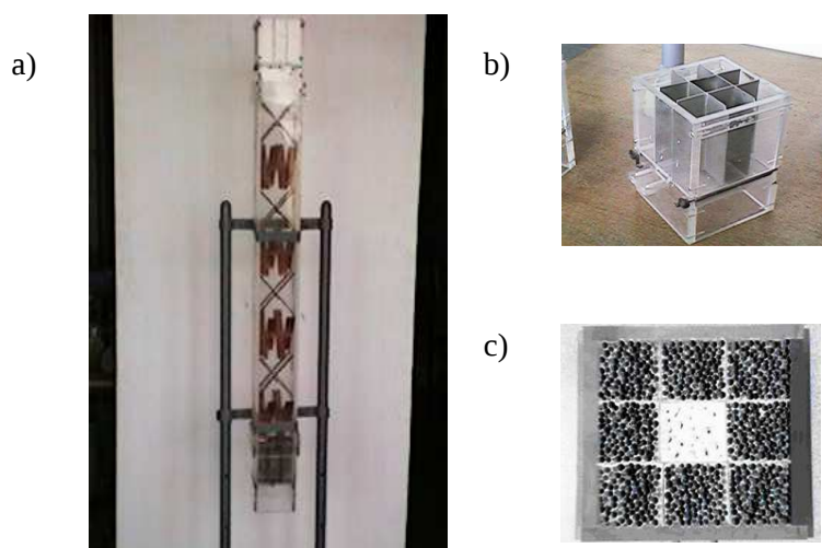
Rys. 1. Mieszalnik statyczny - płytkowy; a) widok ogólny; b) kaseta zasilająca – 9 cel; c) kaseta zasypana materiałem ziarnistym – traser w środkowej celi; (segregacja pierwotna)
