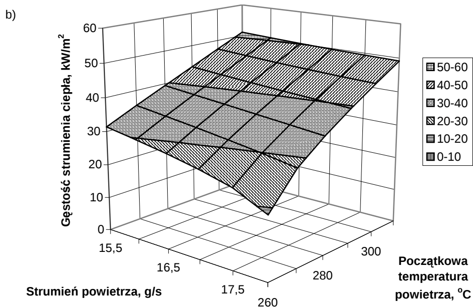
Rys. 2. Wpływ strumienia masy powietrza i jego początkowej temperatury na średnią wartość gęstości strumienia ciepła do nasienia przy strumieniu nasion: a) 0,5; b) 1,0 g/s
