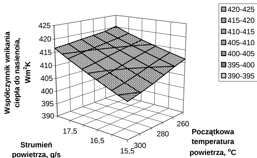
Rys. 1. Wpływ strumienia masy powietrza i jego początkowej temperatury na średnią wartość współczynnika wnikania ciepła do nasienia przy strumieniu nasion: a) 0,5; b) 1,0 g/s
