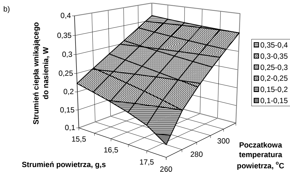
Rys. 3. Wpływ strumienia masy powietrza i jego początkowej temperatury na średnią wartość strumienia ciepła do nasienia przy strumieniu nasion: a) 0,5; b) 1,0 g/s
