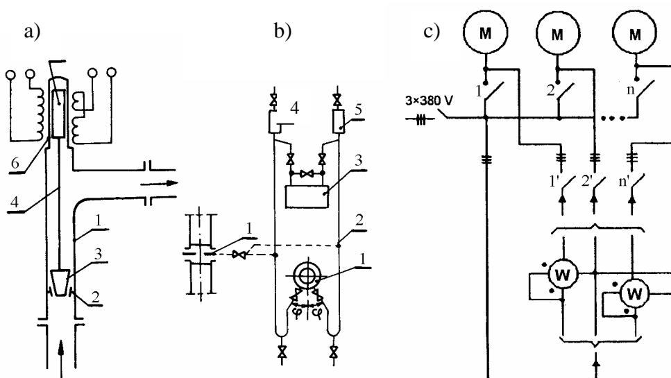
Rys 1. Schematy urządzeń do pomiaru zużycia wody (a), pary wodnej (b), mocy elektrycznej silników (c): a) 1 – obudowa telerotametrów, 2 – zwężka, 3 – pływak, 4 – pręt, 5 – rdzeń ferromagnetyczny, 6 – rura, b) 1 - zwężka pomiarowa (kryza), 2 – przewody impulsowe, 3 – miernik, 4 – odpowietrznik, c) M – trójfazowy silnik indukcyjny, 1, 2, ... , n, 1', 2', ... , n' – styczniki elektromagnetyczne, W – watomierz; watomierz z lewej strony wskazuje moc P_1 , a z prawej – moc P_2
