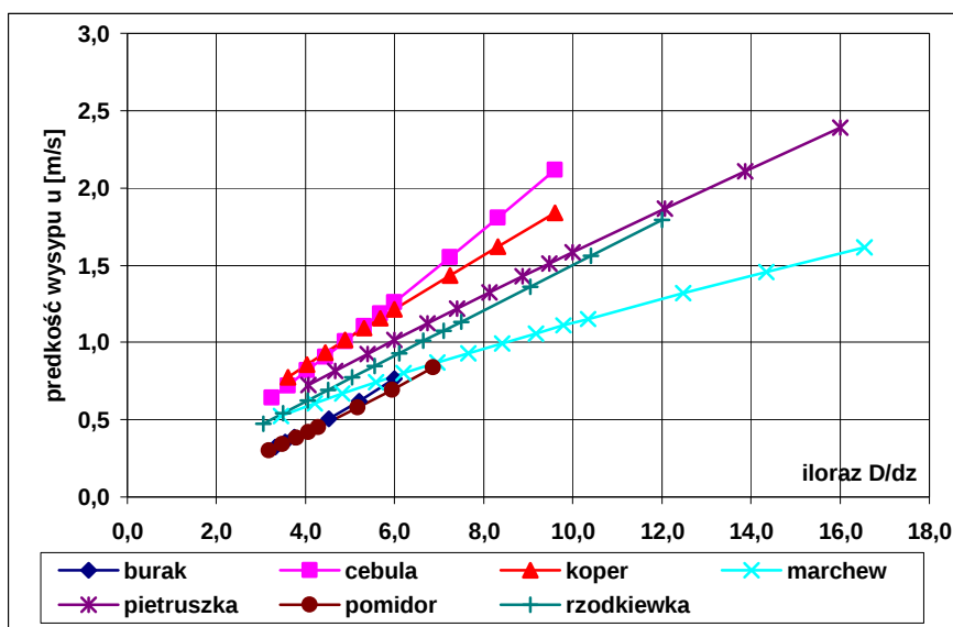
Rys 3. Zależność prędkości wysypu u=f(D/d_{sr}) dla dozownika zamocowanego na kalibratorze.
