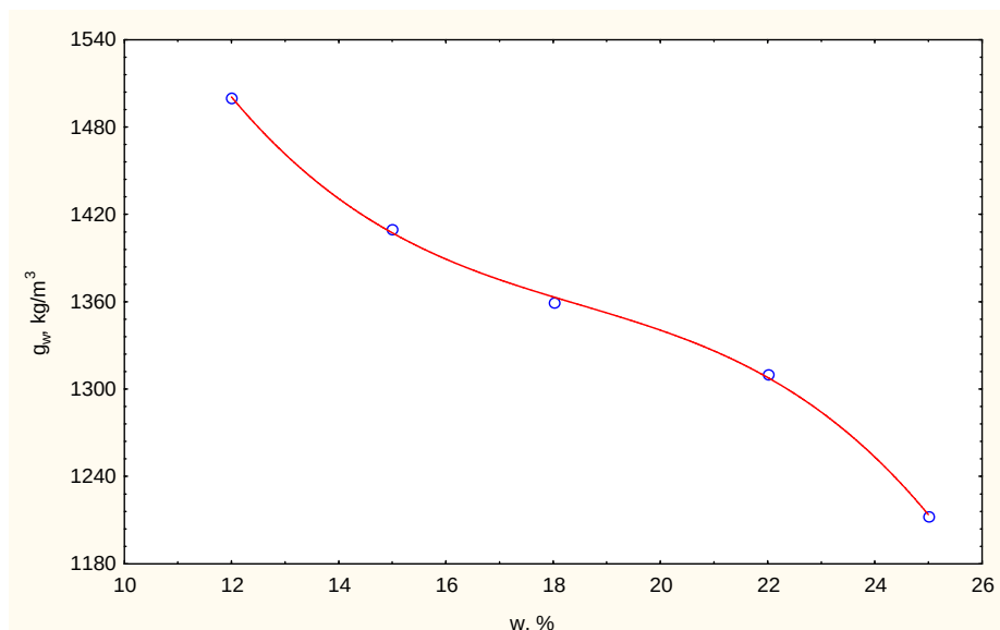
Rys. 1. Wpływ wilgotności nasion łubinu żółtego odmiany Piaś na gęstość właściwą
