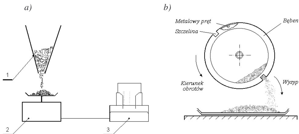
Rys. 1. Zasady pomiaru właściwości reologicznych swobodnie przesypującego się złoży proszku; a) zasada pomiaru indeksu płynięcia, b) zasada pomiaru zdolności płynięcia proszku metodą NIRO; 1 – lejek z kalibrowanym otworem, 2 – waga elektroniczna, 3 - drukarka
