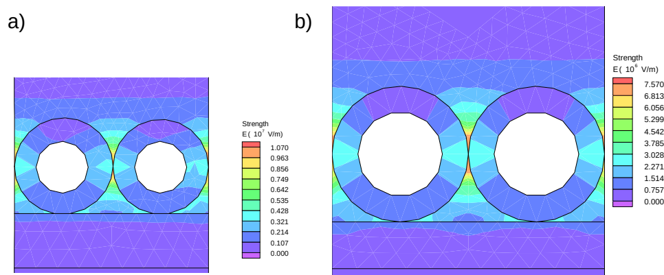
Rys.3. Rozkład natężenia pola elektrycznego wokół uzwojenia bifilarnego wykonanego przewodami o wymiarach: a) d_1 = d_3 = 3,4 \text{ mm} , d_2 = d_4 = 1,8 \text{ mm} , b) d_1 = d_3 = 5,8 \text{ mm} , d_2 = d_4 = 3,6 \text{ mm}
