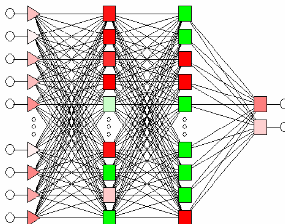
Rys.1 Schemat sieci typu MLP z 2 ukrytymi warstwami
