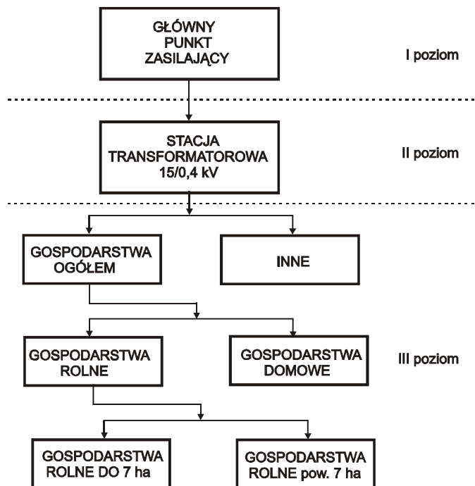
Rys. 1. Podział sieci średniego napięcia na poziomy, a odbiorców na grupy Fig. 1. Division of medium voltage lines into levels and subscribers into groups
