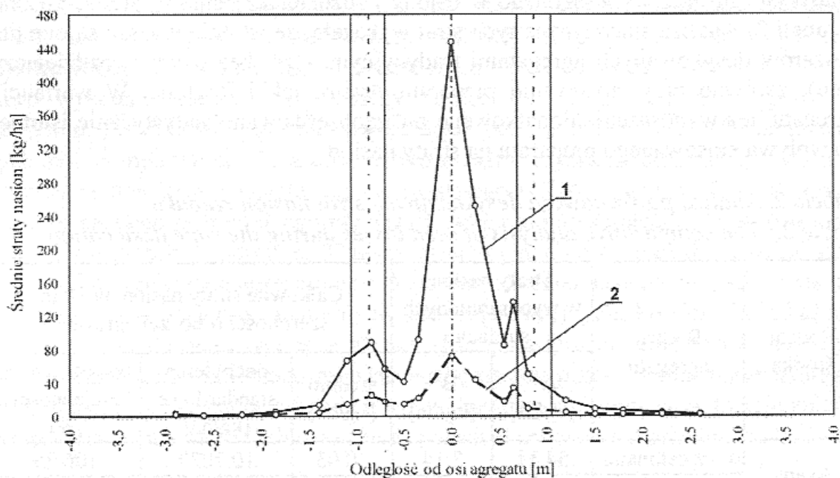
Rys. 2. Średnie straty nasion po zabiegu desykcji rzepaku preparatem Reglone za pomocą agregatu opryskującego wyposażonego w ekran, rozdzielacze łanu i fartuchy osłonowe: 1 – spowodowane osypywaniem się nasion po zabiegu desykcji, 2 – spowodowane zabiegiem desykcji i samoosypywaniem
