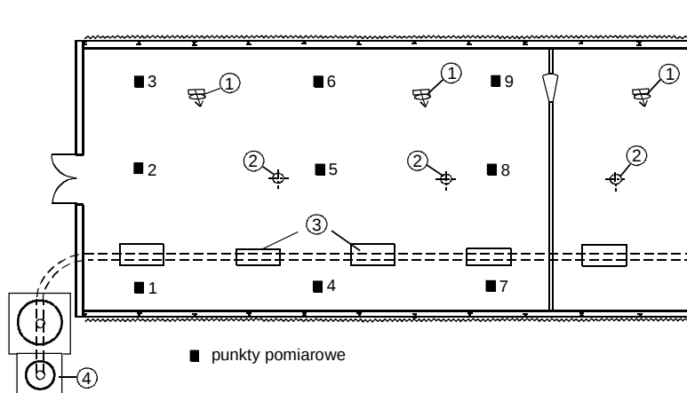
Rys. 1. Rzut przyziemia kojca dla 320 tuczników z rozmieszczeniem punktów pomiarowych. 1 i 2 – wentylatory, 3 - autokarmniki, 4 - silosy na paszę
