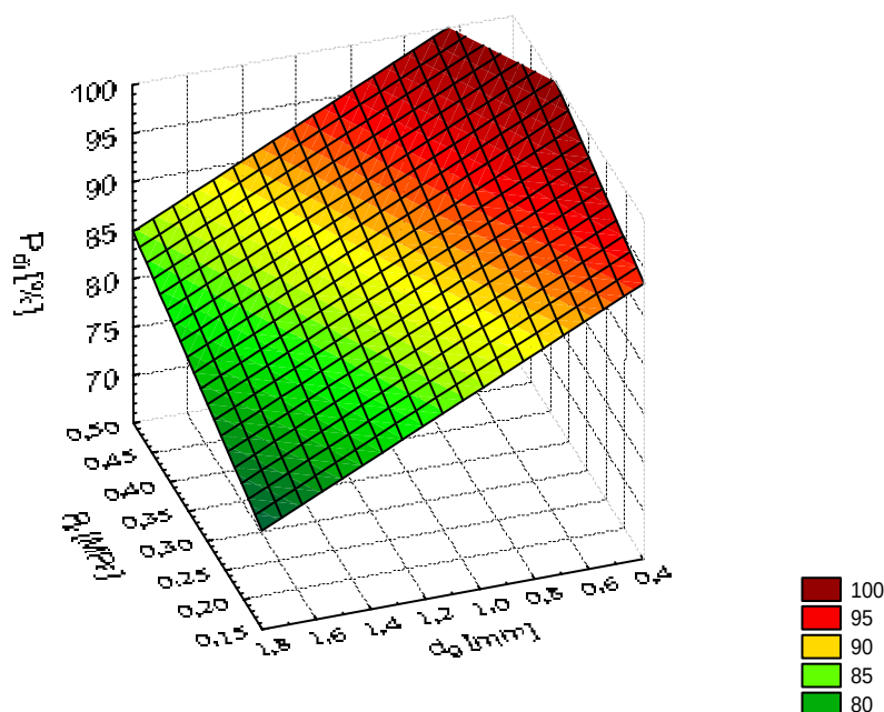
Rys. 1. Zależność pomiędzy wytrzymałością kinetyczną paszy granulowanej a średnicą cząstek granulowanych komponentów i ciśnienia pary podawanej do kondycjonera. Źródło : badania własne.
