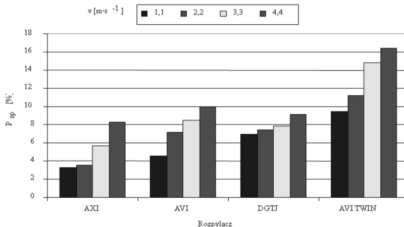
Rysunek 4. Stopień pokrycia powierzchni pionowej najazdowej ( A_{nj} ) dla badanych rozpylaczy Figure 4. Degree of covering the vertical approach surface ( A_{nj} ) for the researched sprayers
