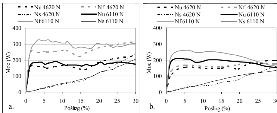
Rysunek 4. Przebiegi mocy składowych w funkcji poślizgu: a) koło z oponą 9.5-24, b) koło z oponą 31x15.5-15 (Nu – moc uciągu, Nf – moc tracona na opór przetaczania, Ns – moc tracona na poślizg)
