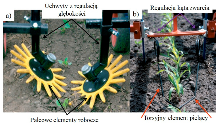
Rysunek 3. Biernie elementy robocze: a) palcowy, b) torsyjny
