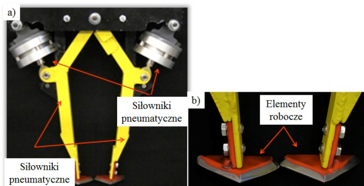
Rysunek 4. Widok narzędzia: a) ramiona wraz z siłownikami pneumatycznymi, b) elementy robocze
