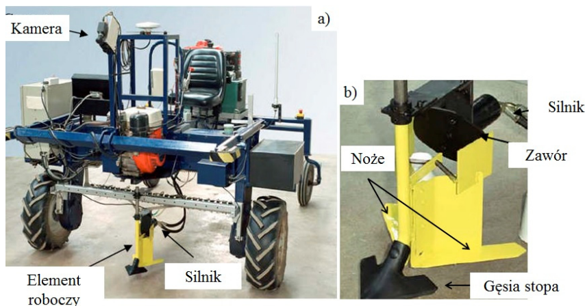
Rysunek 5. Element roboczy z gęsią stópką do zwalczania chwastów w rzędach roślin uprawnych
