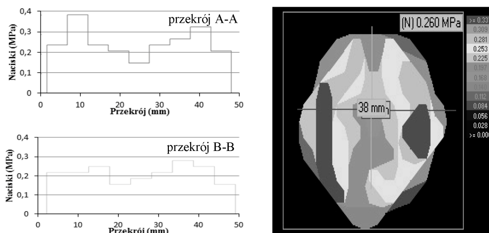
Rysunek 8. Przykładowe warstwicze oraz rozkłady nacisków powierzchniowych, \Delta t = 3 \text{ ms} Figure 8. Exemplary contour lines and distribution of surface pressure, \Delta t = 3 \text{ ms}
