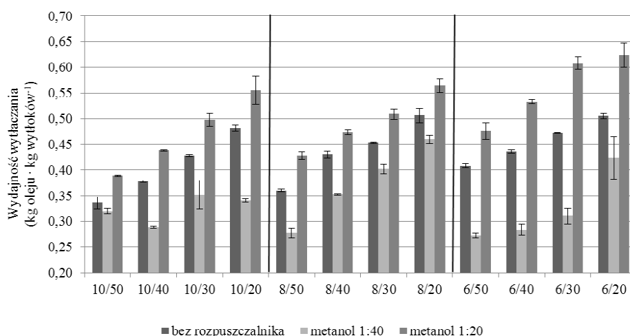
Rysunek 3. Efektywność wyciążania oleju ( \text{kg oleju} \cdot (\text{kg wytłoków})^{-1} ) w zależności od rodzaju obróbki wstępnej, średnicy dyszy prasy oraz obrotów ślimaka prasy Figure 3. Efficiency of pressing oil in ( \text{kg of oil} \cdot (\text{kg of pomace})^{-1} ) depending on the type of initial processing, diameter of the press nozzle and screw rotations
