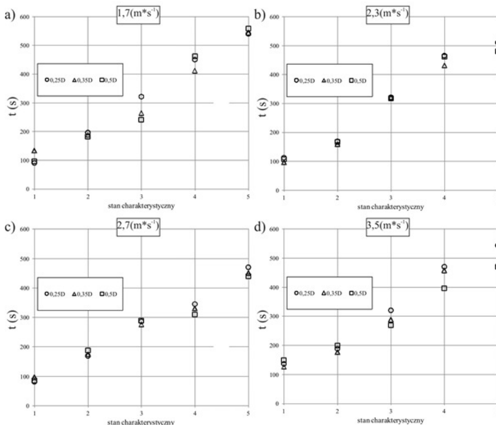
Rysunek 4. Wykresy czasów występowania dla stanów charakterystycznych podczas formowania się stożka osadu w kadzi wirowej (na osi odczytanych wartości jak w rys. 3) dla prędkości napełniania: a) u_{i1}=1,7 m \cdot s^{-1} , b) u_{i2}=2,3 m \cdot s^{-1} , c) u_{i3}=2,7 m \cdot s^{-1} , d) u_{i4}=3,5 m \cdot s^{-1} Figure 4. A plot of timing for the specific formation stages of the sediment cone inside the whirlpool (abscissa: same as pic 3) for the speed of filling a) u_{i1}=1,7 m \cdot s^{-1} , b) u_{i2}=2,3 m \cdot s^{-1} , c) u_{i3}=2,7 m \cdot s^{-1} , d) u_{i4}=3,5 m \cdot s^{-1} Analiza wyników pomiarów czasów występowania
