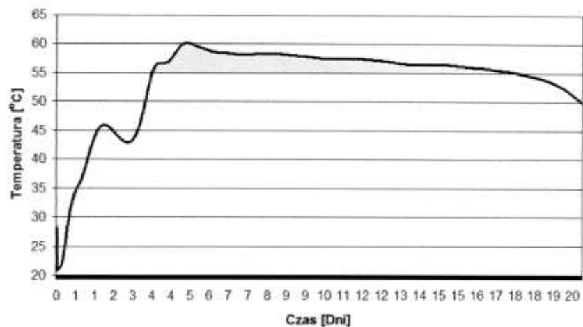
Rys. 2. Przebieg kompostowania pulpy pomidorowej Fig. 2. Course of composting tomato pulp
