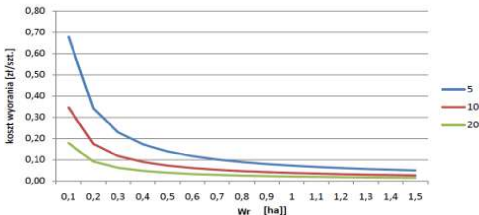
Rys. 2. Koszt jednostkowe wyorywania pojedynczej sadzonki buka zwyczajnego ( Fagus sylvatica L.) wyorywaczem SR 2 w zależności od powierzchni plantacji dla okresu użytkowania maszyny: 5 lat, 10 lat, 20 lat
